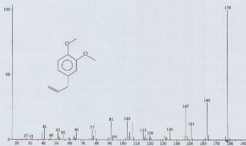
图 A.2 甲基丁香酚标准样品的质谱图
