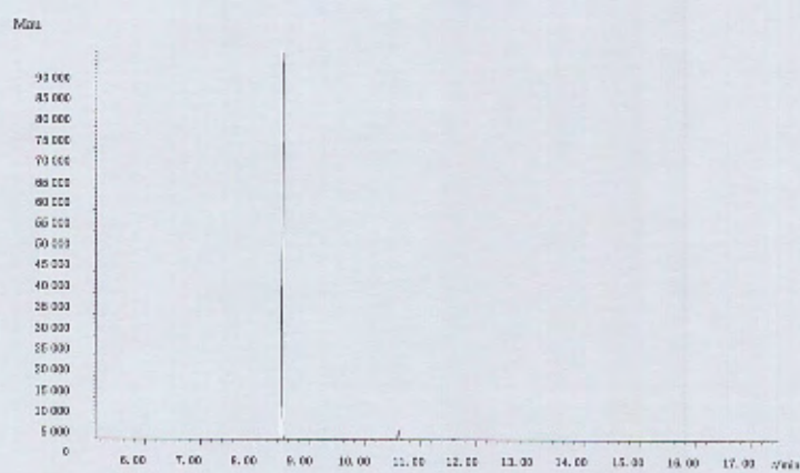
图 A.1 甲基丁香酚标准样品的选择离子监测色谱图
